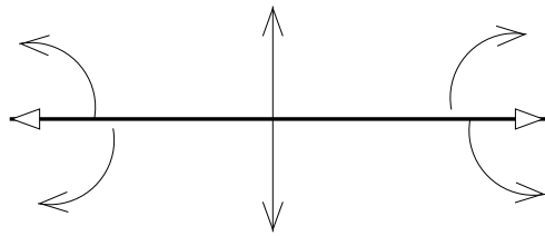
Winged Edge
